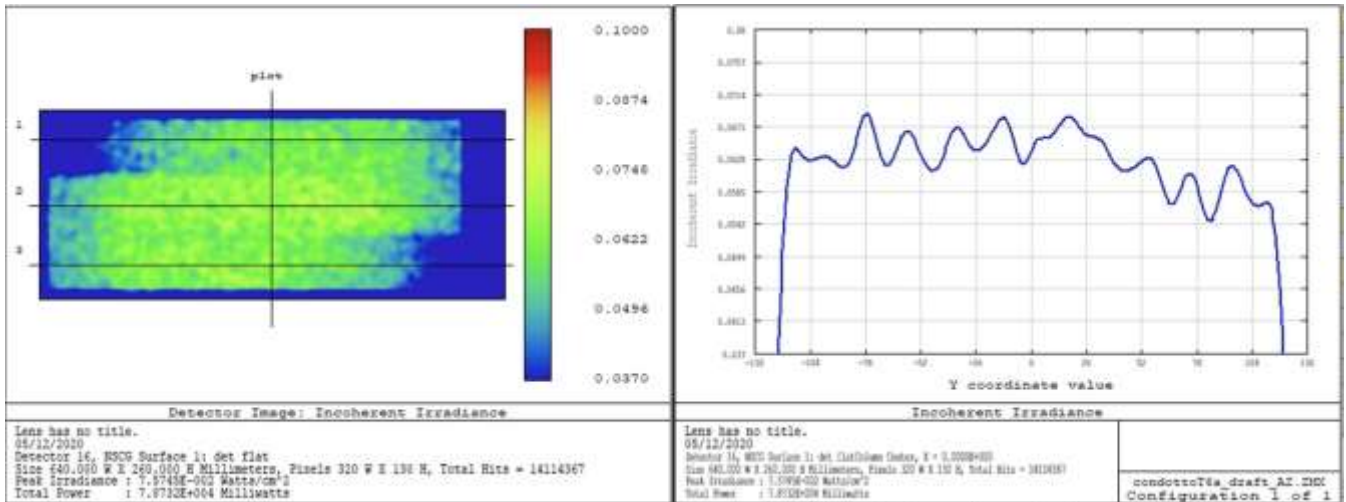
Figura 3: Irradianza (W/cm 2 ) all'interno del canale rilevata dal detector virtuale. E' stato impostato un valore minimo di 0.037 W/cm 2 , in modo da identificare con maggiore facilità le aree sotto soglia (blu). Sono inoltre identificate le sezioni 1, 2, 3 nelle quali sono disposti gli altri detector ortogonali. A destra è riportato il plot cross-section.
