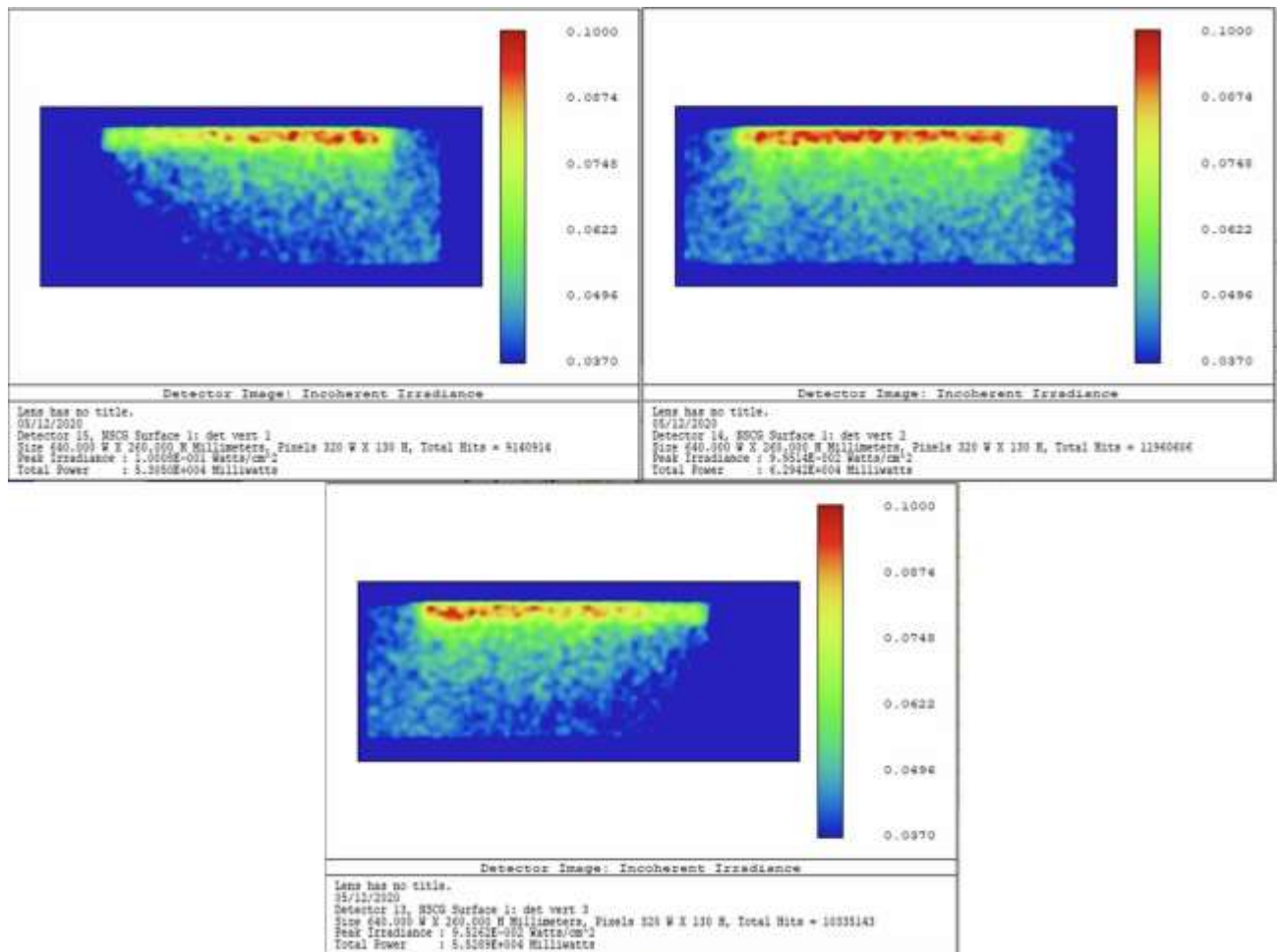
Figura 4: Irradianza (W/cm²) all'interno del canale rilevata dai detector di sezione 1, 2, 3.
